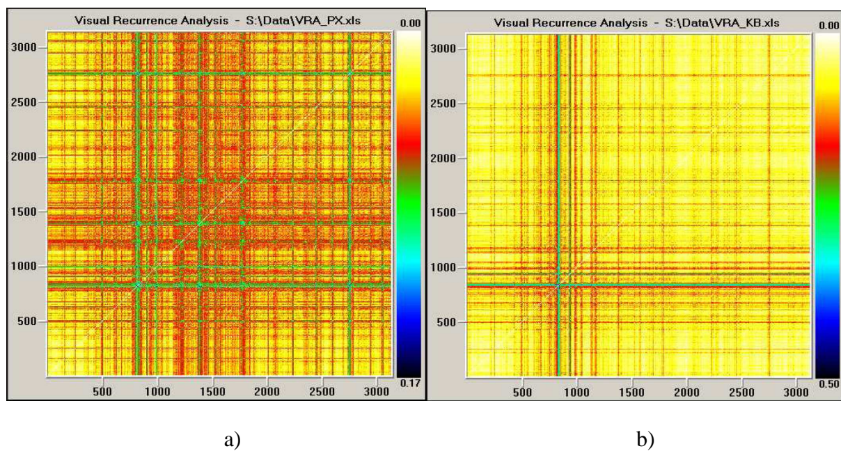
Obr. 5: Rekurenční graf řady výnosností a) akciového indexu PX a b) Komerční banky KB
