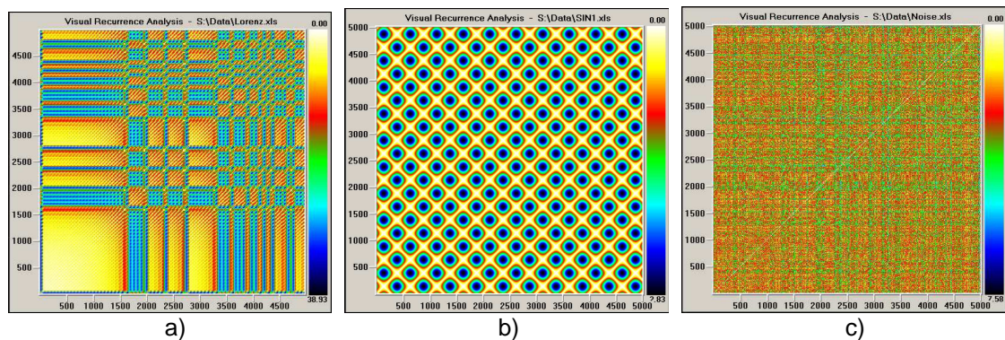
Obr. 1: Rekurenční grafy a) Lorenzova systému, b) periodického sinusoidálního signálu a c) bílého šumu
