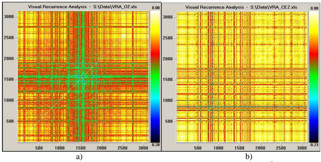
Obr. 8: Rekurenční graf řady výnosností a) akcií Telefonica O2 a b) ČEZu
