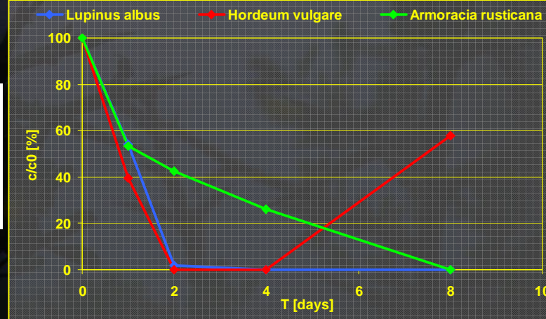
Acetaminofen
