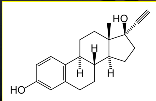
Ethinylestradiol
