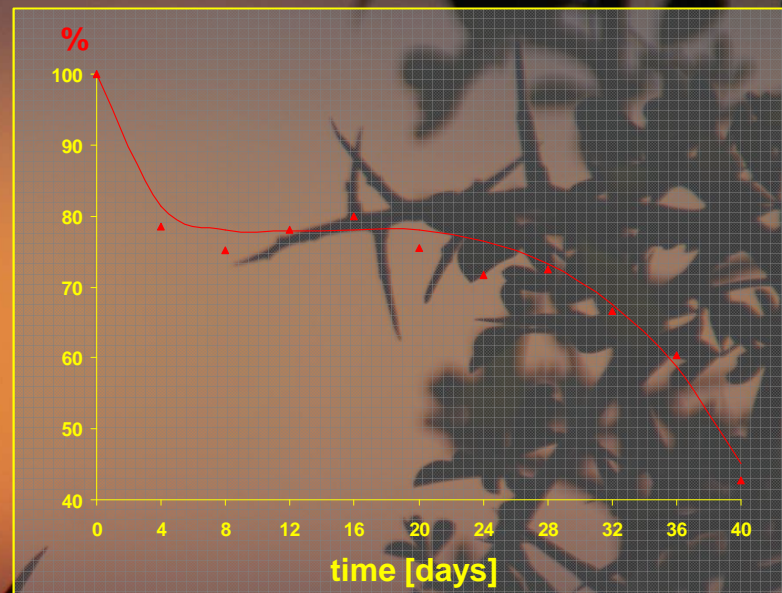
2-chloro-5-nitrobenzene-sulphonic acid
