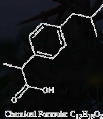
ibuprofen
