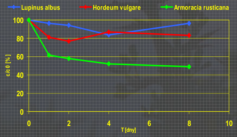
Ibuprofen
