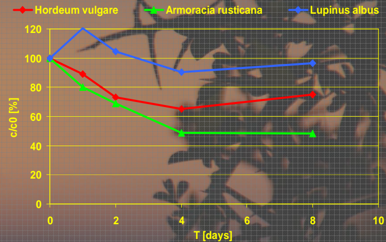
Acetaminofen
