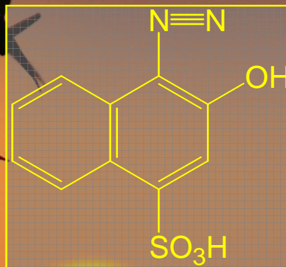
1-diazo-2-naftol-4-sulfonová kyselina
