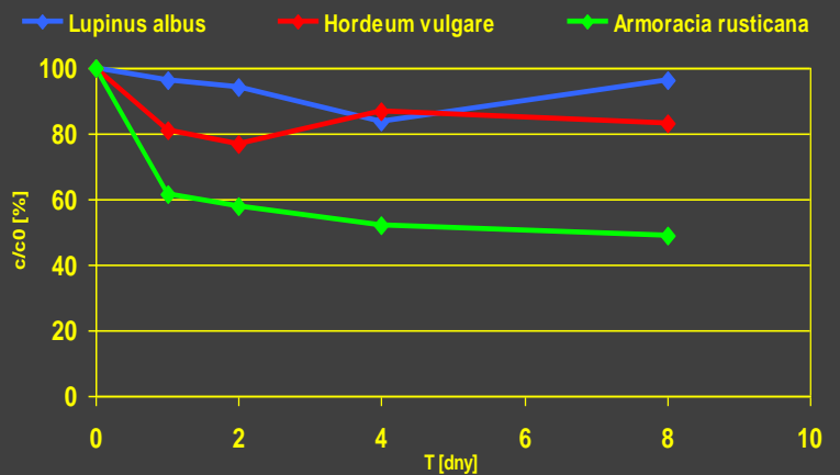
Ibuprofen
