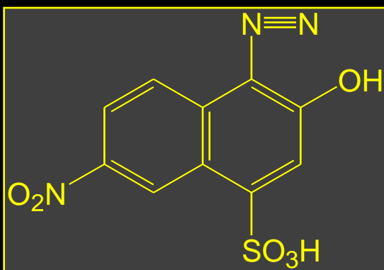
6-nitro-1-diazo-2-naftol-4-sulfonová kyselina
