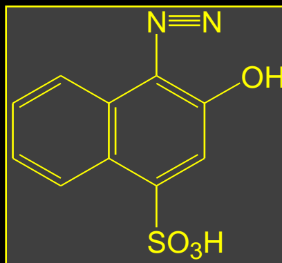
1-diazo-2-naftol-4-sulfonová kyselina
