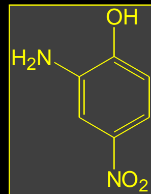
4-nitro-2-aminofenol
