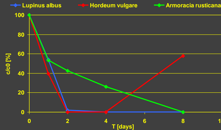
Acetaminofen
