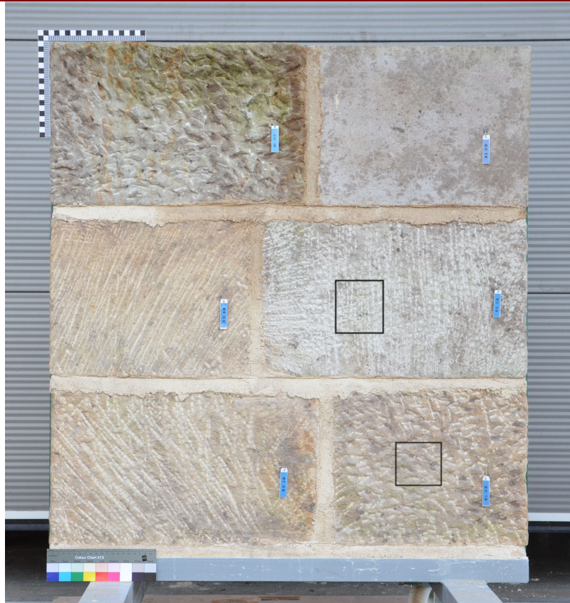
Zkušební bloky s různým způsobem opracování lícních ploch zhotovené pro experimentální potřeby
