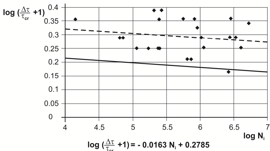
Obr. 1. Křivka únavové pevnosti pro vznik první únavové trhliny
