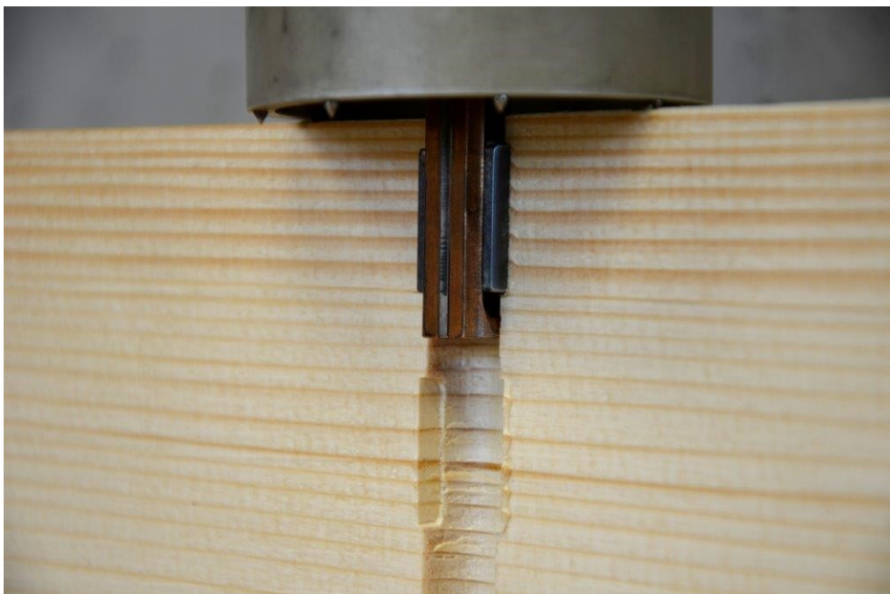
Nová metoda diagnostiky dřeva - roztlačování čelistí ve vrtu
