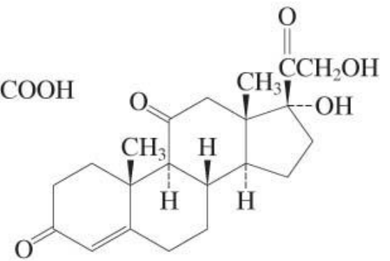
Cortisone
