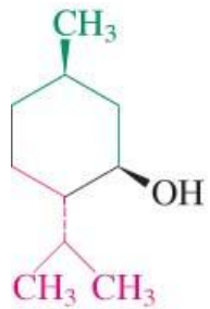
Menthol
