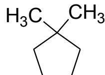
1,1-dimethylcyklopentan
