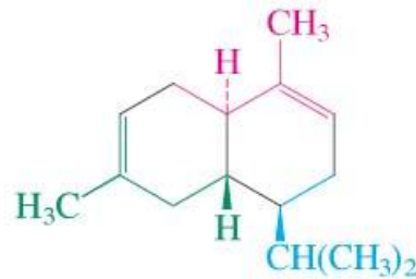
\beta -Cadinene
