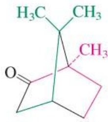
Camphor
