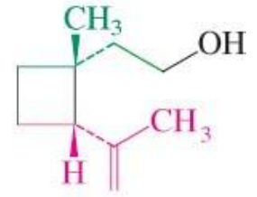
Grandisol
