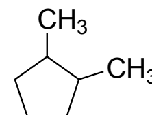
1,2-dimethylcyklopentan
