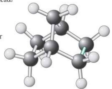
Norbornane
