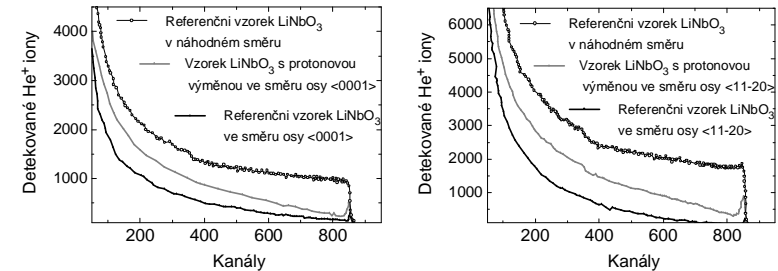
Obr. 15. Srovnání standardního RBS spektra se spektrem ve směru hlavní krystalické osy \text{Er}:\text{LiNbO}_3 a \text{Er}:\text{LiNbO}_3 modifikovaného protonovou výměnou [9].
