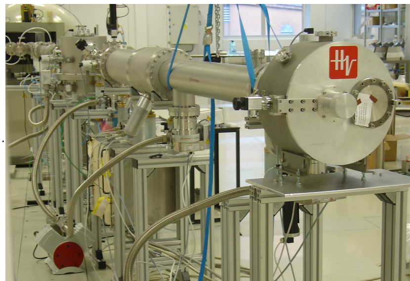
Obr. 2. Implantační iontová trasa
