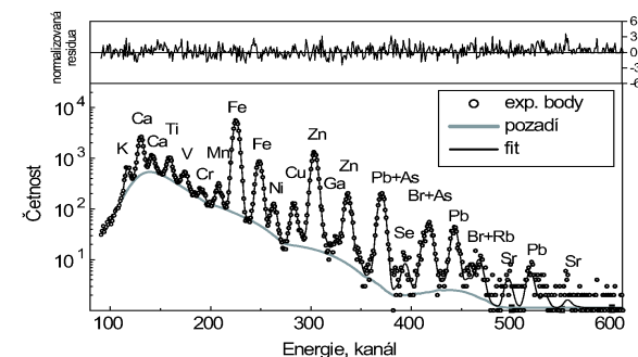
Obr. 10. PIXE spektrum vzorku jemné frakce ( <2.5 \mu\text{m} EAD) atmosférických aerosolů. (2.35 MeV protony, 0,9 mm PE absorbér záření X, fitováno programem PIXE-INP) [4, 6].
