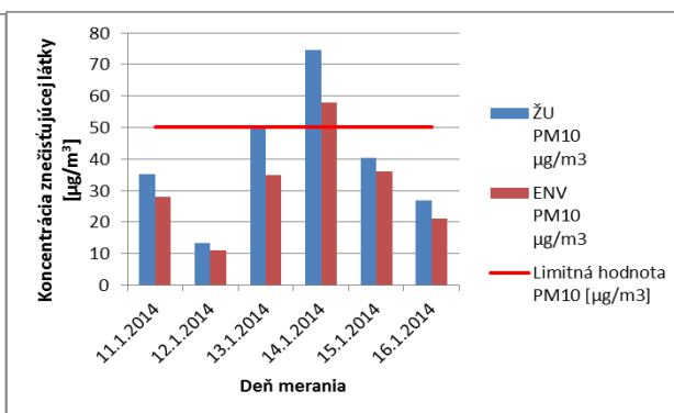
Obr. 4: Porovnanie priemerných denných koncentrácií PM 10 na meracom stanovišti pri diaľnici D1 vo vzdialenosti 7 m (ŽU) a 37 m (ENV) od krajnice CK
