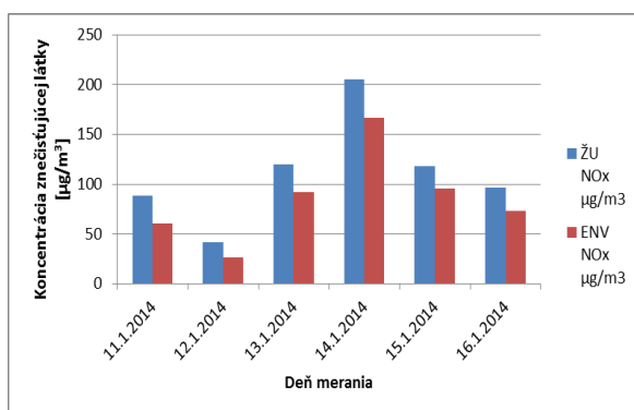
Obr. 3: Porovnanie priemerných denných koncentrácií NO x na meracom stanovišti pri diaľnici D1 vo vzdialenosti 7 m (ŽU) a 37 m (ENV) od krajnice CK
