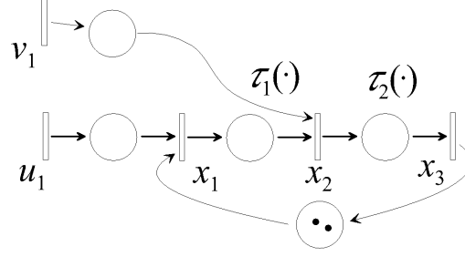
Fig. 1. TEG example.
