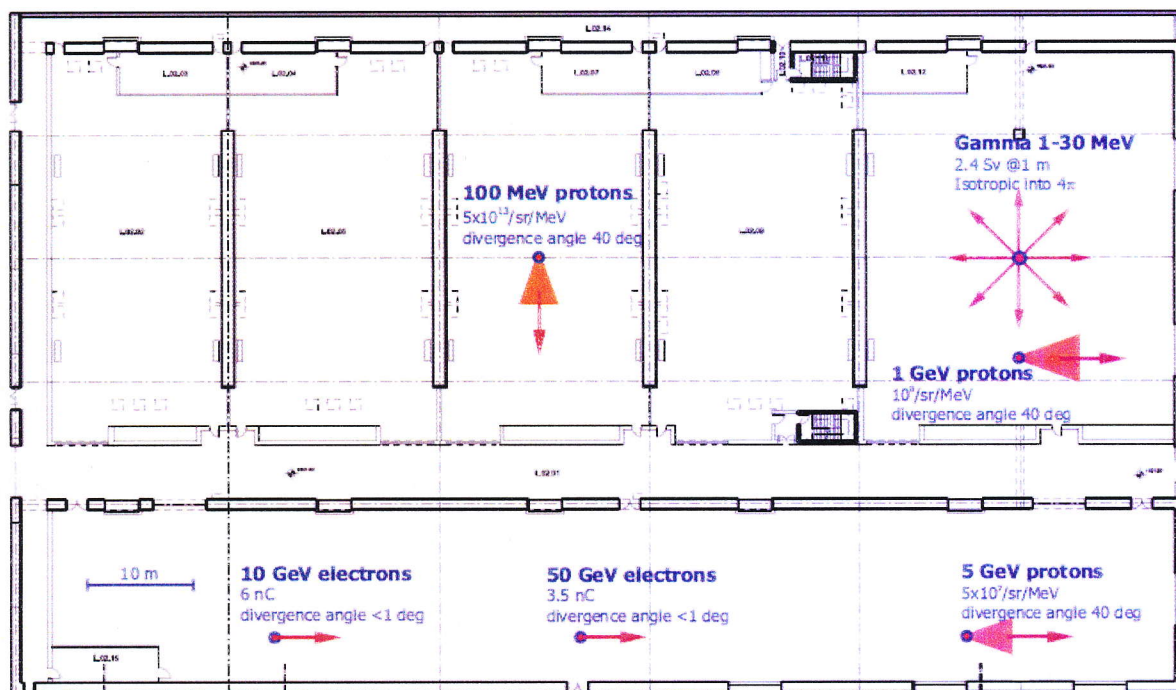
Obr 1. Diagram znázorňující umístění jednotlivých zdrojů a směru jejich vyzařování v podzemním podlaží laserové budovy ELI.
