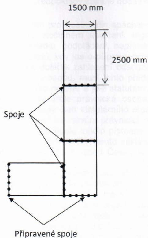
Obrázek: Uspořádání optických stolů.
