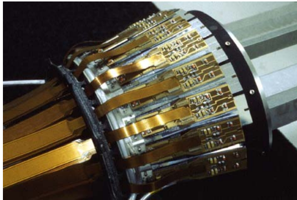
Obr. 7: Pixelový detektor DELPHI vyvinutý ve spolupráci s IHEP ve Vídni
