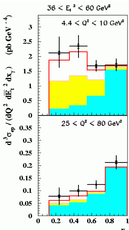
Obr. 10. Účinný průřez pro vznik dvou jetů ve srážce elektronu s protonem pro dva intervaly veličiny Q^2 . Modrý plný histogram představuje předpověď teorie bez započtení efektů struktury fotonu, červená čára po jejich započtení.
