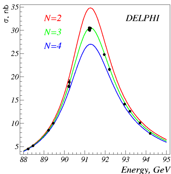
Obr. 6: Závislost účinného průřezu anihilace elektronů s pozitrony na hadrony dokazující, že existují právě jen tři generace fundamentálních fermionů.
