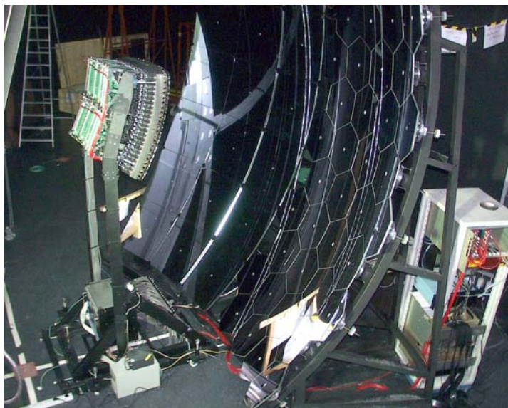
Obr.18 Zrcadla pro Observatoř Pierra Augera vyrobená v SLO.
