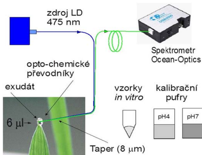
Obr. 2. Vláknově-optická detekce biologických vzorků o malých objemech
