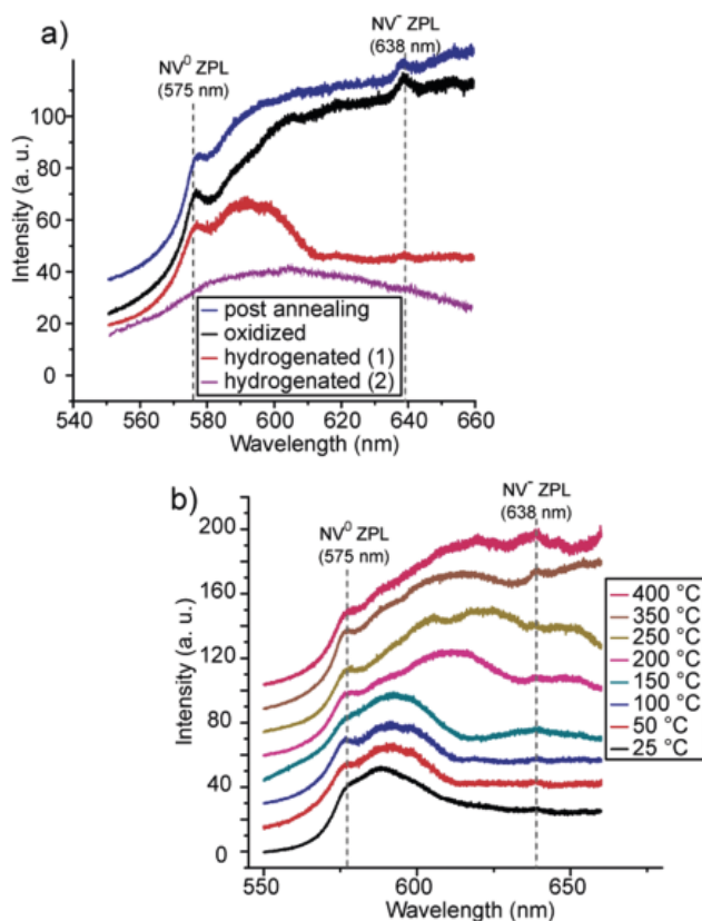
■ Obr. 12 Luminiscenční spektra oxidovaných, vodíkem terminovaných a následně žíháných diamantových zrn: žíhání při 400 °C vede k obnově původní povrchové terminace (kyslíkové), resp. původní luminiscenční odezvy. Terminace zrn o velikostech ~40 nm vodíkem vedla k posuvu, resp. k vyhasínání luminiscence NV - center a pro velmi malé částice (< 20 nm), luminiscence NV - center vyhasla kompletně.
