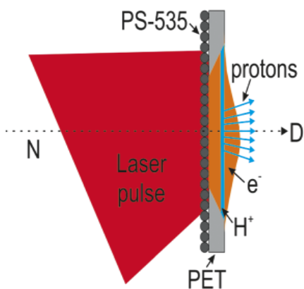
Vlevo: Mechanismus TNSA se speciální geometrií terče použitou v experimentu (boční pohled). Laserové záření se absorbuje na rozhraní nanokuliček a vakua, kam dopadá pod úhlem 22,5°. Horké elektrony (generované na přední straně terče) prolétávají terčem a urychlují protony na jeho zadní straně. Vpravo: energetické spektrum urychlených protonů pro různé průměry nanokuliček na terči.
