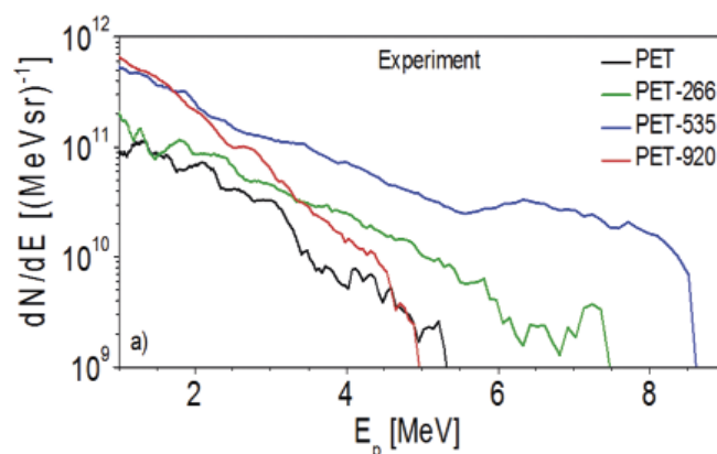
Vlevo: Mechanismus TNSA se speciální geometrií terče použitou v experimentu (boční pohled). Laserové záření se absorbuje na rozhraní nanokuliček a vakua, kam dopadá pod úhlem 22,5°. Horké elektrony (generované na přední straně terče) prolétávají terčem a urychlují protony na jeho zadní straně. Vpravo: energetické spektrum urychlených protonů pro různé průměry nanokuliček na terči.
