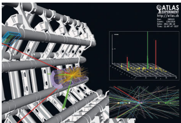
■ Obr. 1 Rozpad Higgsova bosonu H \rightarrow \mu^+ \mu^- e^+ e^- , jako ho registrovala aparatura ATLAS. Červeně jsou zobrazeny dráhy mionů, zeleně dráhy elektronů a pozitronů. V pravém dolním rohu je zobrazena série protonových srážek, při jejichž identifikaci a správném přiřazení drah vzniklých částic má nezastupitelnou roli pixelový detektor.
