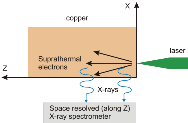
■ Obr. 11 Ozařování masivní mědi femtosekundovými laserovými pulsy poblíž přesně definované hrany terčů (vlevo) poskytuje prostřednictvím zobrazovací rentgenové spektroskopie informace o generaci a šíření horkých elektronů (vpravo)
