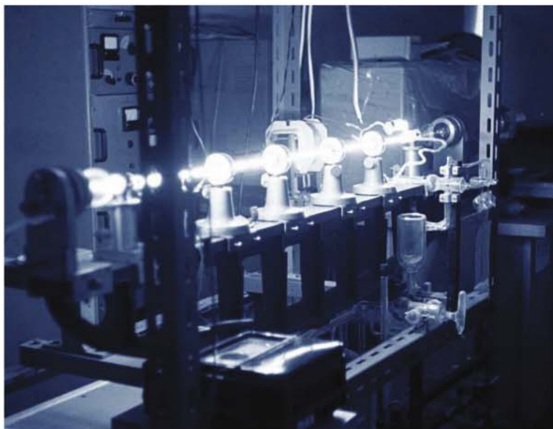
Obr. 12 Kadmiový laser generující modré koherentní záření 441,6 nm (ÚRE-ČSAV 1970).
