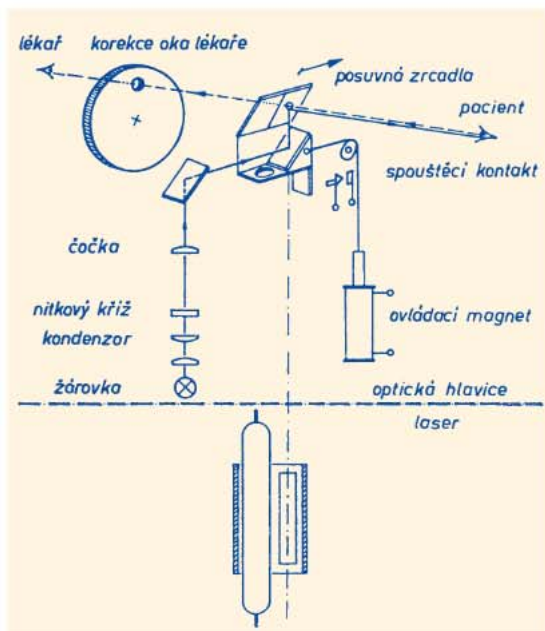
Obr. 8 Schematické uspořádání optické hlavičky kvantového koagulatoru – kombinace upraveného oftalmoskopu s miniaturním rubínovým laserem.
