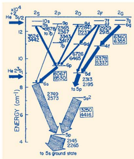
Obr. 11 Mechanismus excitace kadmia srážkami s heliem na vyšší energetické hladiny CdII (podle [42]). (Pevné čáry – excitace ionty He + , šrafované plochy – excitace Penningovou reakcí, vlnové délky uzavřené v hranatém boxu reprezentují kontinuální režim.)
