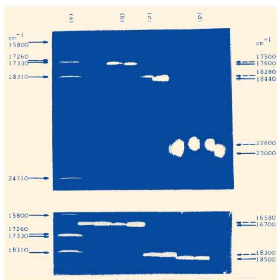
Obr. 13 Spektra impulzního barvivového laseru. Koncentrace barviv: 5 \times 10^{-3} mol/l (plné čáry), 1 \times 10^{-3} mol/l (přerušované čáry); (a) kalibrační čáry, (b) rhodamin 6G, (c) Na-fluorescein, (d) coumarin 120, (e) rhodamin B [46].
