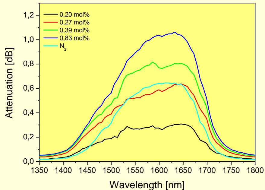
Toluen (g)
