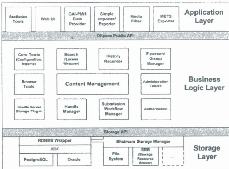
Fig. 1. DSpace layers
