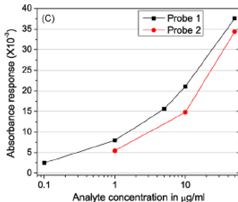
Kalibrační křivky
