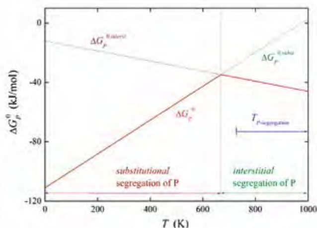
Obr. 11 Teplotní závislost Gibbsovy energie segregace fosforu v Fe, \Delta G_p^0 . Vínová tečkovaná čára v levé části obrázku je konstruována pro experimentální data s intersticiální segregací fosforu. Zelená tečkovaná čára je založena na teoretických výsledcích a odpovídající entropie odhadnuta podle modelu Lejčka a Hofmanna pro substituční segregaci. Plná červená čára ukazuje minimální hodnotu \Delta G_p^0 při teplotách 0–1000 K. Svíslá tečkovaná čára označuje „transformační“ teplotu, T_{tr} , mezi substituční a intersticiální segregací fosforu. Oblast označená modrou šipkou reprezentuje teploty experimentálního studia segregace fosforu na hranicích zrn.
