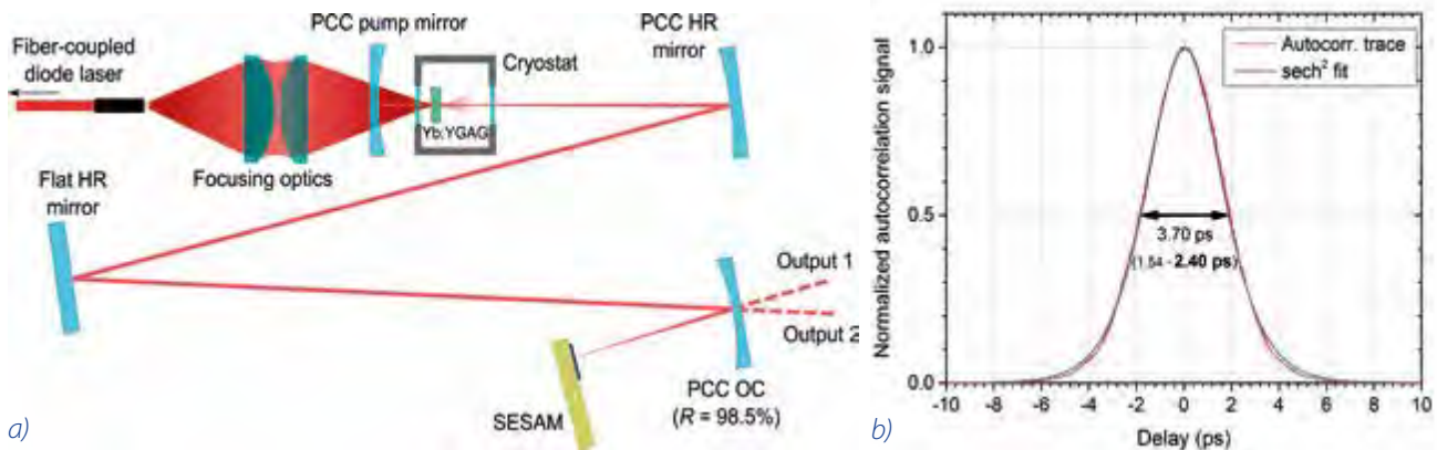
Obr. 6 (a) Optické schéma kryogenně chlazeného Yb:YAG laserového oscilátoru se synchronizací módů pomocí polovodičového saturovatelného absorbéru; (b) intenzitní autokorelace vygenerovaných pulsů odpovídá 2,4 ps dlouhým \text{sech}^2 pulsům.
