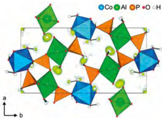
■ Obr. 4 Struktura hlinitofosforečnanu kobaltnatého překrytá mapou diferenčního elektrostatičeského potenciálu (žluté isopovrchy). Mapa jednoznačně ukazuje pozice atomů vodíku ve struktuře.
