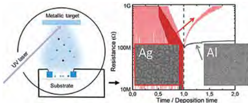
■ Obr. 5 Měření in-situ rezistivity Ag/Al a příprava plazmonových struktur pro zesílení luminescence.
