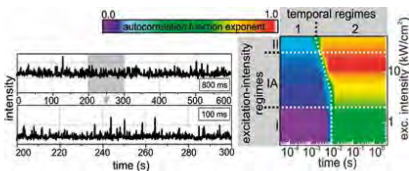
■ Obr. 15 Dynamika blikání křemíkových nanokrystalů. Nalevo: příklad pozorovaného blikání (nahore), spodní panel ukazuje vybraný časový interval ve větším rozlišení. Napravo: tento graf shrnuje pozorované typy chování za různých experimentálních podmínek v rámci popisu pomocí autokorelační funkce. Lze nalézt režimy s i bez závislosti na excitační intenzitě.
