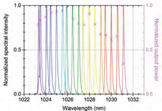
■ Obr. 5 Přeladitelnost kryogenně chlazeného Yb:YAG aktivního prostředí měřená pomocí dvojlovných filtrů v CW režimu.
