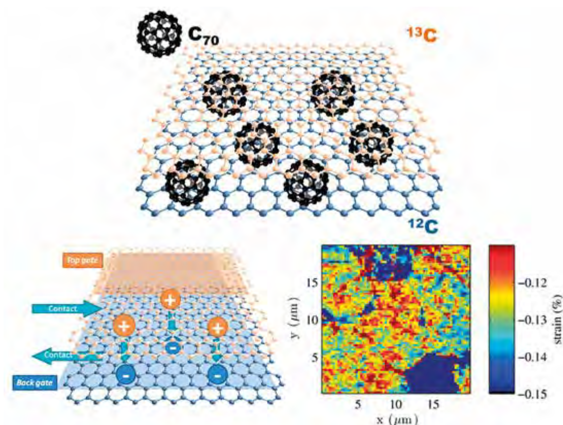
Struktura dvojdímenzionálního analugu fullerenového lusu na bázi \text{C}_{70} s izotopově značenými monovrstvami grafenu. Vlevo dole je schematicky znázorněna architektura BiSFET, vpravo dole mapa distribuce mechanického napětí horní vrstvy grafenu určená na základě experimentu Ramanovské mikrospektroskopie.
