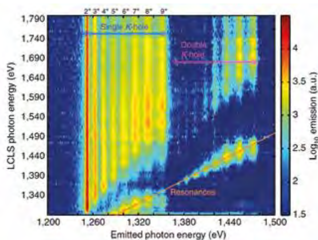
■ Obr. 12 Emisní spektrum izochoricky ohřátého hořčíku zobrazující polohy Ka hran. Vodorovná osa udává energii emitovaných Ka fotonů a svislá osa je energie FEL fotonů.
