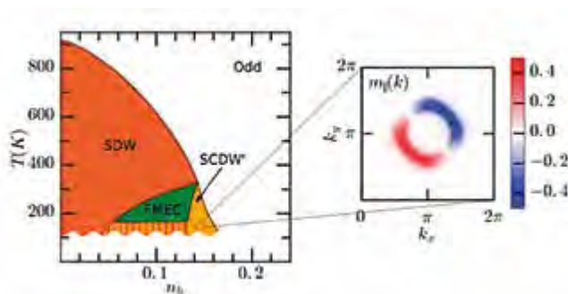
Termodynamické fáze studovaného modelu v závislosti na teplotě ( T ) a počtu elektronů na atom ( 2-n_b ). Barevné oblasti odpovídají různým druhům excitonového kondenzátu. Fáze označená SCDW vykazuje spinovou texturu, viz pravý panel zobrazující distribuci magnetizace v Brillouinově zóně.
