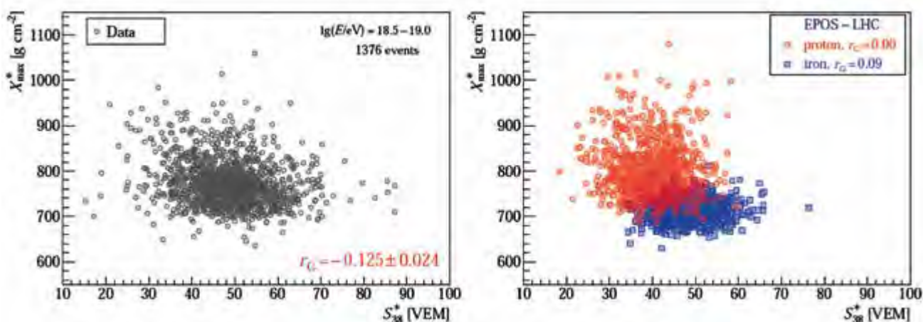
■ Obr. 2 Vlevo závislost hloubky maxima spršky v atmosféře měřená fluorescenčním detektorem na velikosti signálu v povrchovém detektoru (reálná data). Vpravo simulace stejných veličin pro protony a jádra železa pomocí modelu EPOS-LHC. Podrobným kvantifikováním korelací těchto dvou veličin bylo prokázáno smíšené složení kosmického záření v oblasti kotníku spektra kosmického záření [14].
