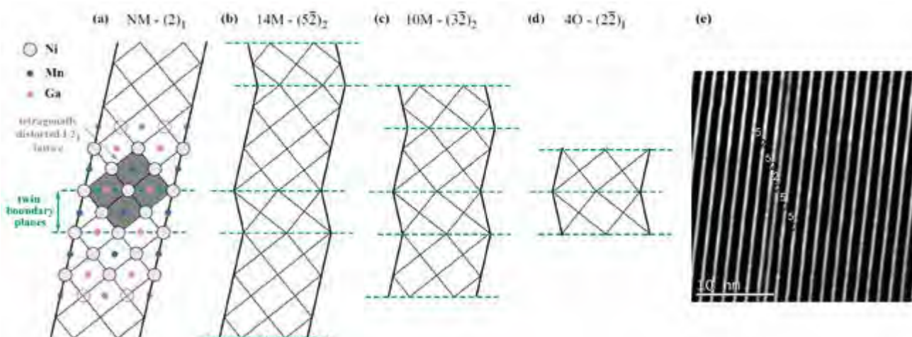
■ Obr. 9 Schematická ilustrace nanotwinovaných martensitických struktur v Ni 2 MnGa slitinách s magnetickou tvarovou pamětí a) základní struktura NM, b) 14M neboli (52) struktura, c) 10M neboli (32) struktura, d) předpovězená 4O neboli (22) struktura, e) experimentální pozorování 4O struktury (222..) stacking v lokálním (atomovém) měřítku.
