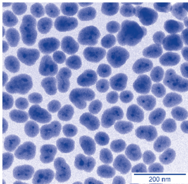
■ Obr. 10 Snímek z transmisní elektronové mikroskopie ukazující klastry nanočástic feritu \text{Mn}_{0,61}\text{Zn}_{0,42}\text{Fe}_{1,97}\text{O}_4 obalené amorfním hydratovaným oxidem křemičitým.
