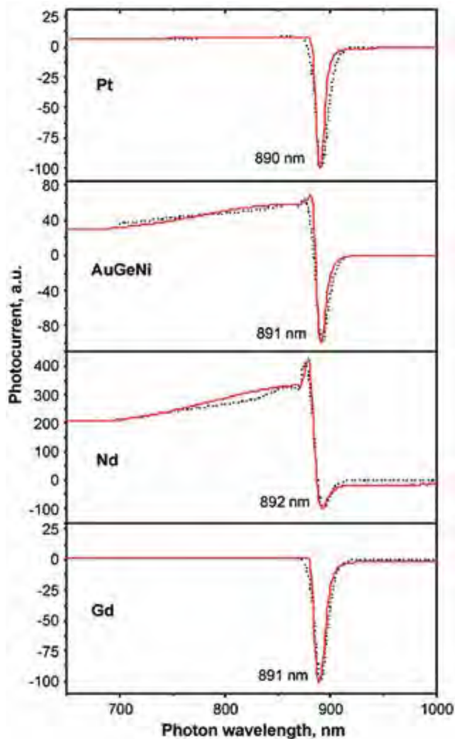
■ Obr. 2 Spektrální závislost fotoproudu měřeného nakrátko pro detektorové struktury na bázi Si-GaAs s různými typy semitrparentního pokovení. Červené spojité křivky odpovídají experimentu, černé křivky simulaci. (Převzato z [2])
