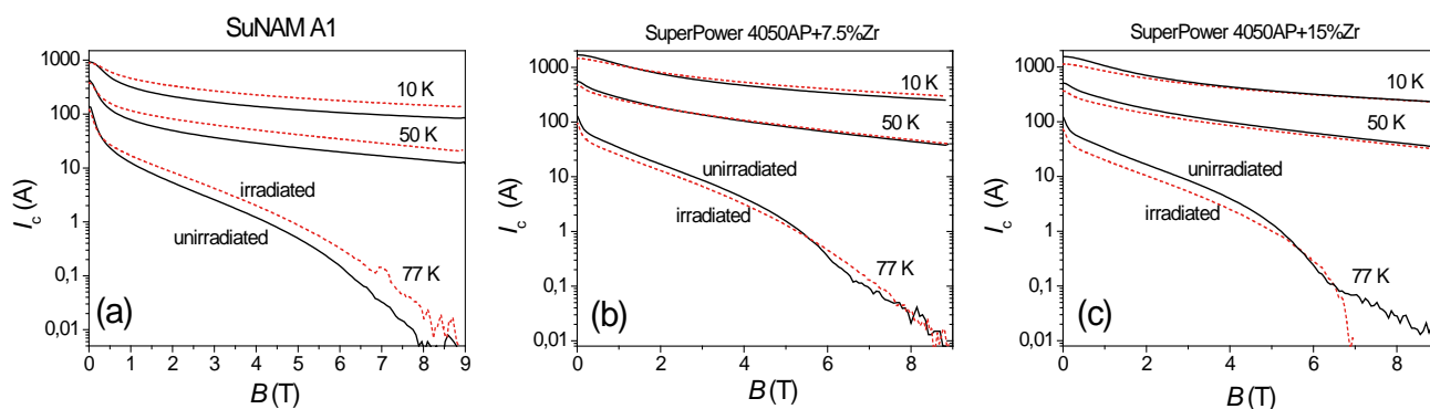
Obr. 18 Vliv ozáření neutrony na jmenovitý proud páskou. Dávka neutronového ozáření byla 2,1 \cdot 10^{22} \text{ m}^{-2} . (a) Páska SuNAM A1, (b) páska SuperPower dopovaná 7,5 % Zr, a (c) páska SuperPower SCS 4050AP dopovaná 15 % Zr.
