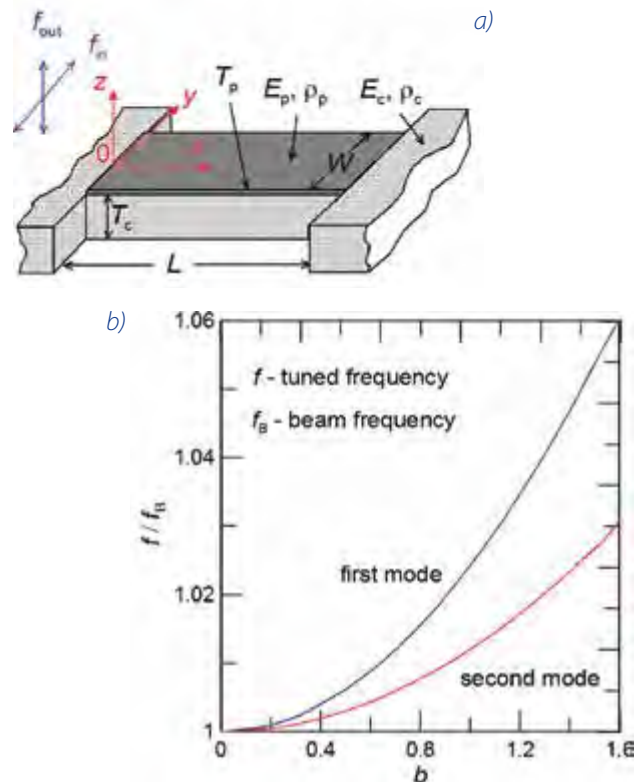
■ Obr. 7 a) Ilustrace uvažovaného oboustranně vetknutého nosníku z elastického substrátu pokrytého tenkou vrstvou, b) obecná závislost rezonanční frekvence na tahovém parametru b pro první dvě rezonanční frekvence.
