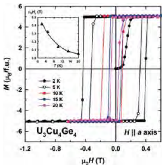
Obr. 12 Anizotropní konstanty a hysteretní smyčky U_3Cu_4Ge_4 v různých teplotách.
