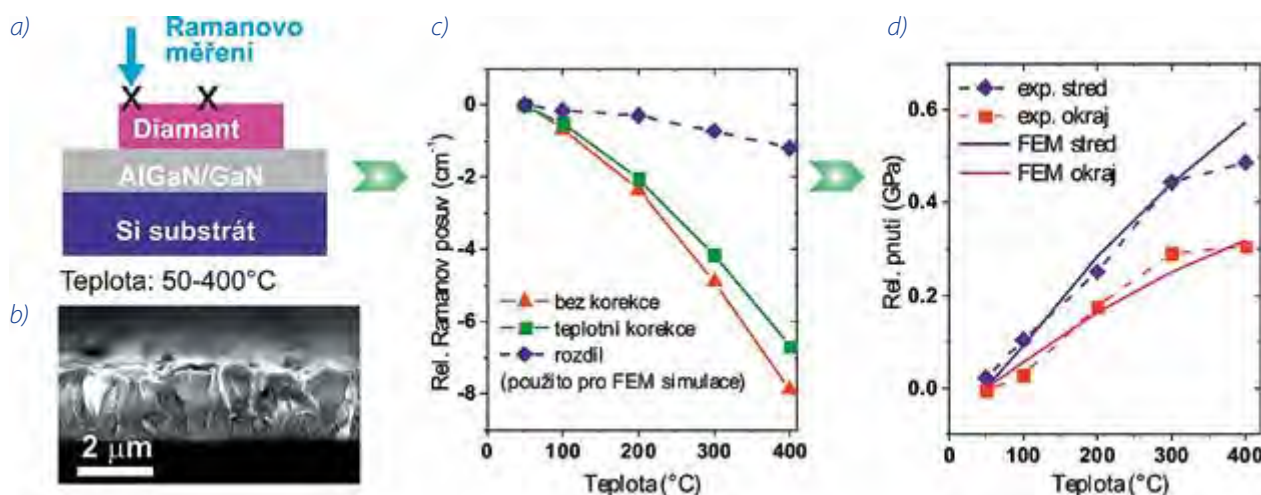
■ Obr. 23 (a) Schematické zobrazení řezu a (b) morfologie heterostrukury diamant-AlGaN/GaN. Grafická závislost (c) teplotně korigovaného Ramanova posuvu diamantového maxima heterostrukury diamant-AlGaN/GaN a teplotně indukovaného pnutí vztaženého k teplotě 50°C.
