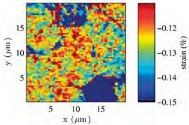
■ Obr. 13 Struktura dvojdimenzionálního analoga fullerenného lusu s izotopově značenými monovrstvami grafenu (vlevo) a mapa distribuce mechanického napětí horní vrstvy grafenu určená na základě analýzy Ramansky aktivních módů grafenu (vpravo).
