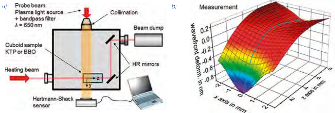
■ Obr. 3 (a) Optické schéma měření deformace optických krystalů zahříváných optickým svazkem pomocí měření vlnoplochy příčného referenčního svazku; (b) změřená deformace vlnoplochy referenčního svazku v krystalu KTP – k největší deformaci dochází v oblasti AR vrstvy (fialově).
