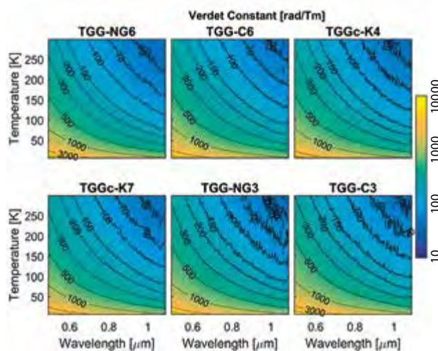
■ Obr. 10 Grafické znázornění Verdetovy konstanty vybraných TGG materiálů pro různé teploty a vlnové délky.
