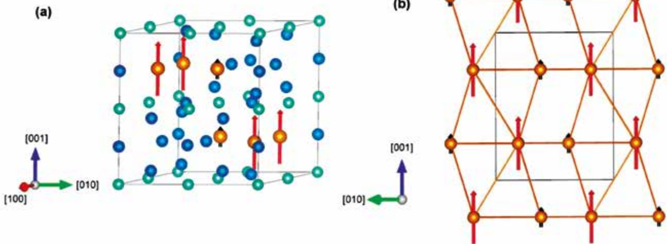
■ Obr. 6 Feromagnetická struktura Nd_3Ru_4Al_{12} při teplotě 2 K. Magnetické momenty jsou vyznačeny šipkami. Barevný kód: (Nd: oranžová; Ru: modrozelená; Al: modrá).
