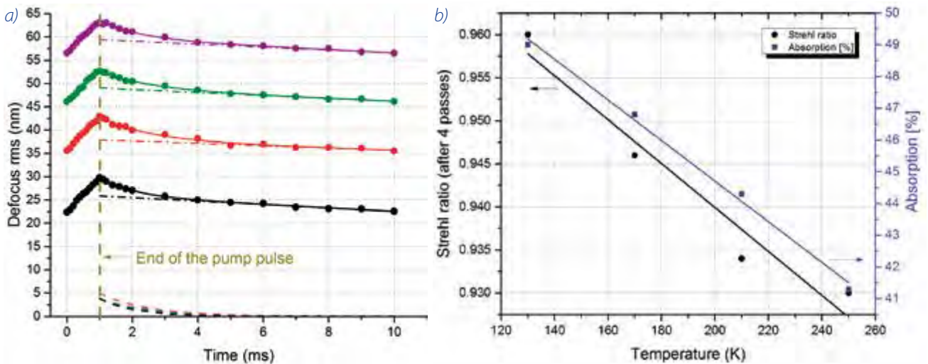
■ Obr. 4 (a) Klesající optická aberace (defokus) s klesající teplotou aktivního prostředí při buzení aktivního prostředí 1 ms dlouhým pulsem s vlnovou délkou 940 nm (černě 130 K, fialově 250 K). Čárkovaně vyznačen vliv změny indexu lomu díky excitaci elektronů. (b) Klesající vliv optických aberací na kvalitu laserového svazku po zesílení v multiprůchodovém kryogenně chlazeném zesilovači.
