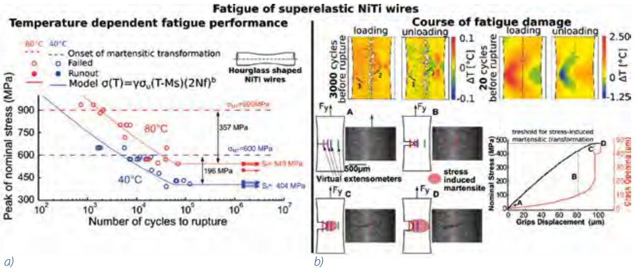
■ Obr. 6 Únavové vlastnosti superelastických slitin NiTi a) únavová křivka maximální napětí – počet cyklů do lomu, b) detekce lokalizované transformace pomocí IR kamery.
