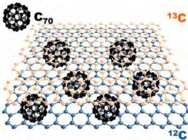
■ Obr. 13 Struktura dvojdimenzionálního analoga fullerenného lusu s izotopově značenými monovrstvami grafenu (vlevo) a mapa distribuce mechanického napětí horní vrstvy grafenu určená na základě analýzy Ramansky aktivních módů grafenu (vpravo).
