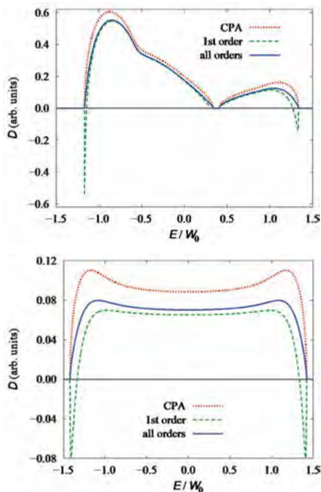
■ Obr. 16 Nahoře: Difusní konstanta pro binární slitinu s komponentní koncentrací 30 % – 70 % a s rozdílem atomových potenciálů komponent \Delta V = W_0 , kde 2W_0 je šířka energetického pásu čistého homogenní krystalické mřížky. Dole: Podobná konfigurace pro spojitě rozložené hodnoty náhodného potenciálu na intervalu (-W_0, W_0) . Jednotlivé křivky odpovídají výpočtu s přiblížením koherentního potenciálu (CPA), prvního řádu započtení vrcholových korekcí (1st order) a pro poruchovou řadu sečtenou do všech řádů na jednoduše kubické krystalické mřížce.
