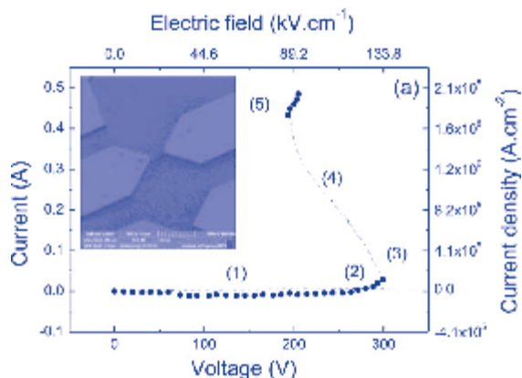
■ Obr 10 a) Quasi-statická voltampérová charakteristika 22,4 μm dlouhého borem dopovaného diamantového testovaného zařízení, která vykazuje (1) lineární ohmickou oblast při nízkém elektrickém poli, (2) nelineární nosičem zesílenou oblast, (3) kritické napětí způsobené lavinovou ionizací neutrálních příměsí, (4) přechodovou oblast s negativním odporem, a (5) oblast vysoké vodivosti. (Detail: obrázek testovaného zařízení pořízený rastrovacím elektronovým mikroskopem). b) Experimentálně určená závislost průrazného napětí na mezelektrodové vzdálenosti pro různé koncentrace akceptorů (tečkovaně). Pro srovnání jsou uvedeny Paschenova křivka (čárkovaně) a modifikovaná Paschenova křivka (tečkovaně), obě identifikované na vzduchu, a dále je pro srovnání zobrazen spodní limit průrazného napětí nedopovaného diamantu (intenzita průrazného pole cca 1\text{ MV cm}^{-1} ).
