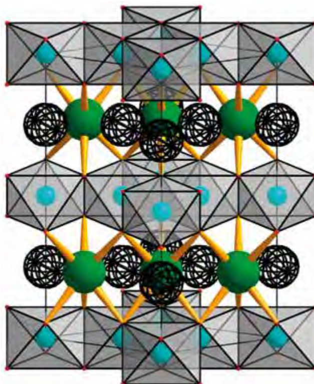
■ Obr. 8 Základní strukturní blok superstruktury \text{Ln}_x\text{CoO}_2 ( \text{Ln} = \text{La}, \text{Pr} a \text{Nd} , x \sim 1/3 ). Ionty Ln obsazují 1/3 poloh (zelené plné kuličky), které jsou pravidelně uspořádány s 2/3 vakantních poloh (černé síťované kuličky). Ionty kobaltu (modré plné kuličky) jsou zobrazeny společně se svým koordinacním okolím.
