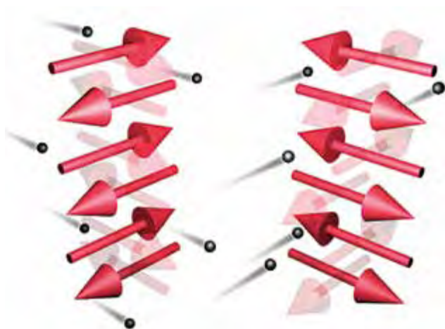
■ Obr. 3 Převzato ze sekce Insights/Perspectives časopisu Science z doprovodného článku „Addressing an antiferromagnetic memory“ k naší publikaci [7]. Na ilustraci proud elektronů (černé kuličky) přepíná směr antiferomagnetických momentů (červené šipky).
