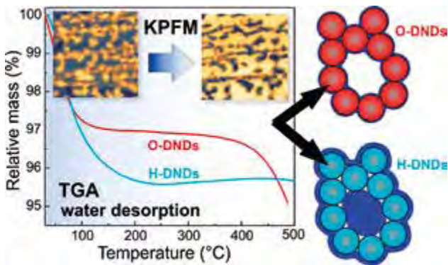
■ Obr. 17 Termogravimetrická analýza pro hydrogenované (modře) a oxidované (červeně) detonační nanodiamanty. V horní části grafu jsou ukázány KPFM skeny hydrogenovaných nanodiamantů s adsorbovanou povrchovou vodou (vlevo) a po desorpci povrchové vody (vpravo), znázorněné na modelu v pravé části obrázku.
