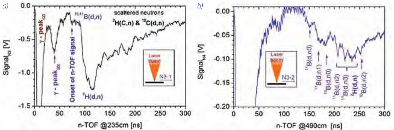
■ Obr. 14 Signály scintilačních detektorů N3-1 (a) a N3-2 (b) umístěných ve vzdálenostech 235 a 490 cm od terčíku ozářeného laserovým systémem PALS [25]. První dva píky zaznamenané během prvních 70 ns jsou odezvou na gama záblesky. Další píky odpovídají neutronům generovaným v důsledku fúze deuteronů s bórem, uhlíkem a deuterony.
