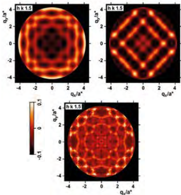
■ Obr. 16 Počítačová simulace anomálního difuzního rozptylu na krystalu \text{SrTiO}_3 pro model I (vlevo) a model II (uprostřed) a její porovnání s experimentálně naměřenými hodnotami (vpravo). Obraz anomálního difuzního rozptylu byl získán jako rozdíl intenzit difuzního rozptylu pro energie fotonů 15,50 keV a 16,09 keV, tj. pro energie s různým příspěvkem anomálního rozptylu od atomů stroncia. Upraveno podle [26].
