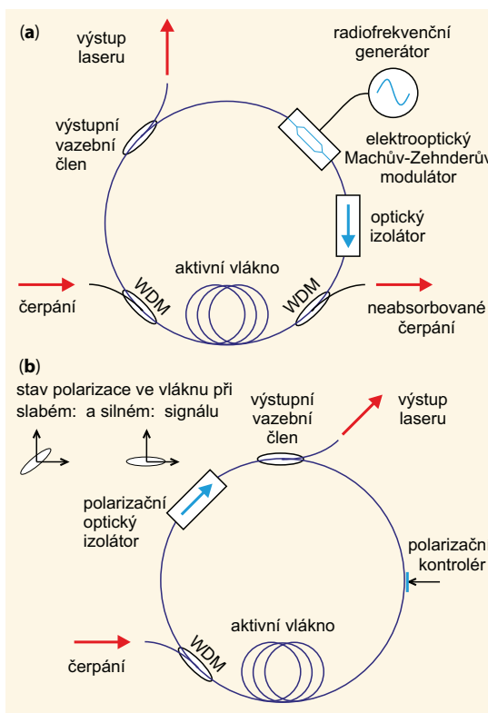
Obr. 2 Příklady uspořádání pulsního vláknového laseru s aktivní (a) a pasivní (b) módovou synchronizací.
