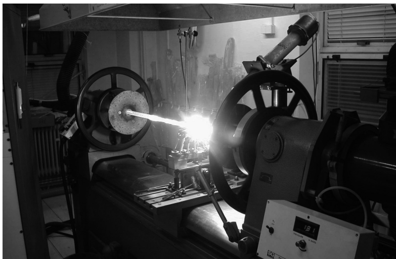
Obr. 3. Příprava preformy optického vlákna na sklářském soustruhu s kyslíko-vodíkovým hořákem v laboratoři technologie optických vláken Ústavu fotoniky a elektroniky AV ČR, v.v.i.
