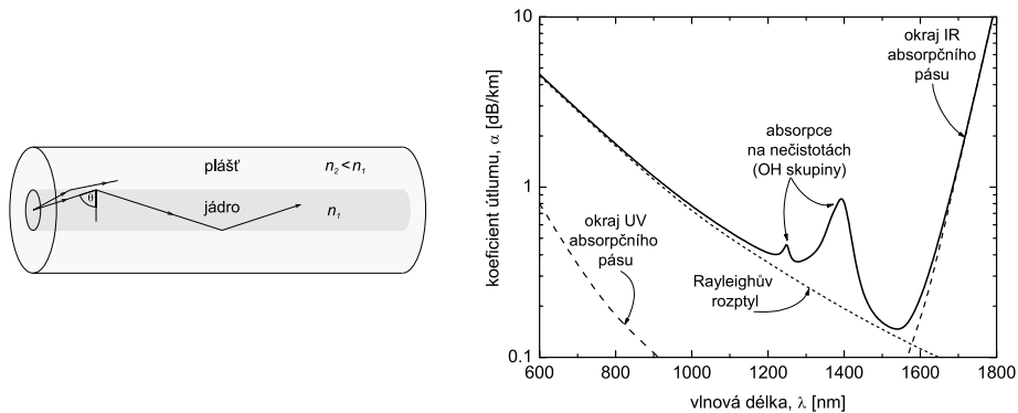
Obr. 2. Struktura optického vlákna (vlevo). Optické vlákno, které je jednomódové na vlnových délkách 1300 nm i 1550 nm, má typicky průměr jádra 8 \mu\text{m} a průměr křemenného pláště 125 \mu\text{m} . Křemenné vlákno je ještě pokrýváno polymerní ochrannou vrstvou a má celkový průměr 0,25 \text{ mm} . Spektrální závislost útlumu optického vlákna z křemenného skla (vpravo).
