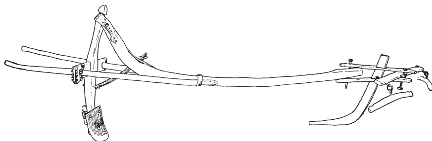
Krkonošský (slezský, orlický, trutnovský) hák s botkovým chodáčkem, krpadly a s váhou s rozporkami. Lomnice n. Popelkou
