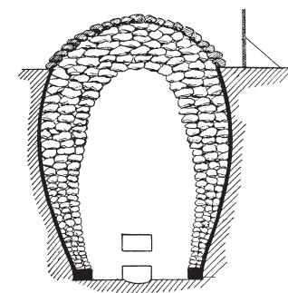
Průřez malou vápenic. Lažánky u Tišnova, 1960
