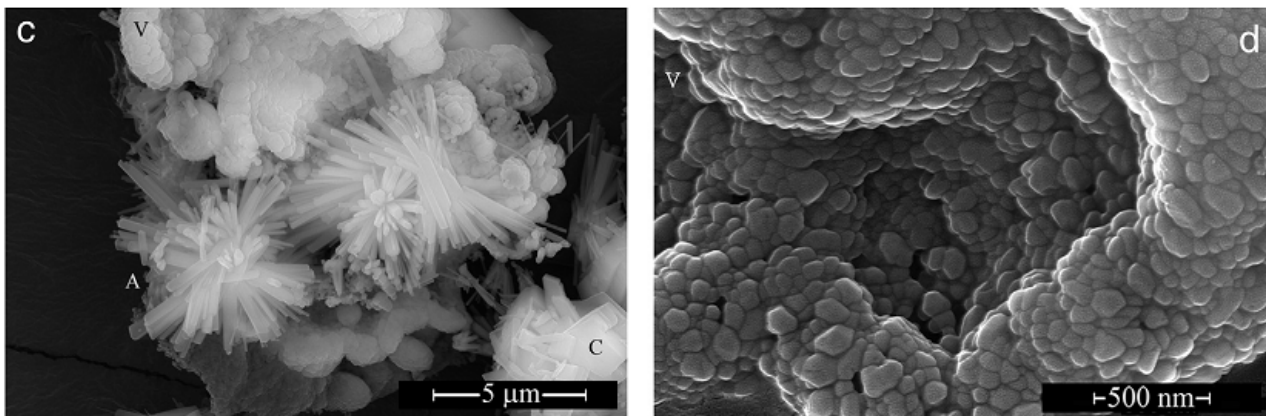
SEM fotografie vateritu syntetizovaného při různých teplotách (a – T = 30^{\circ}\text{C} , 600 ot/min; b – T = 60^{\circ}\text{C} , 600 ot/min; c – T = 90^{\circ}\text{C} , 600 ot/min). SEM fotografie nanostruktury vateritu (d – T = 60^{\circ}\text{C} , 600 ot/min). Polymorfy \text{CaCO}_3 jsou označeny (V = vaterite, C = calcite, A = aragonite).
