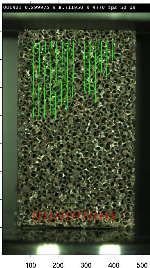
Impaktní test hliníkové pěny vyplněné polymerem
