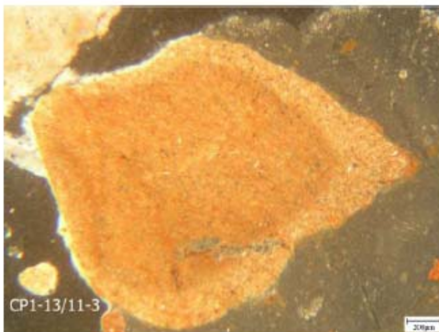
Mikroskopický snímek cihlového úlomku v maltě - Struktura povrchu úlomku cihly s reakčním lemem různé tloušťky (RPL), zvětšeno 500×, měřítko = 200 µm
