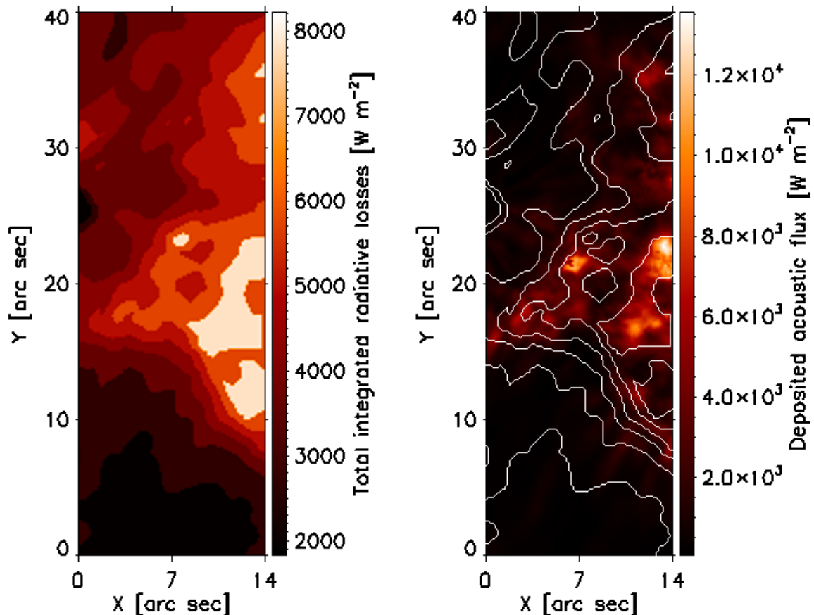
Obr. 2: Mapy malé části slunečního povrchu ( 10 \text{ Mm} \times 29 \text{ Mm} ) ve srovnávaných veličinách. Vlevo zářivé ztráty, vpravo tok energie zvukových vln spolu s obrysy z mapy zářivých ztrát.
