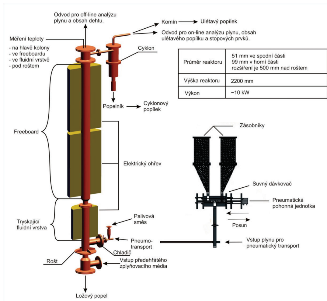
Fluidní zplyňovací generátor
