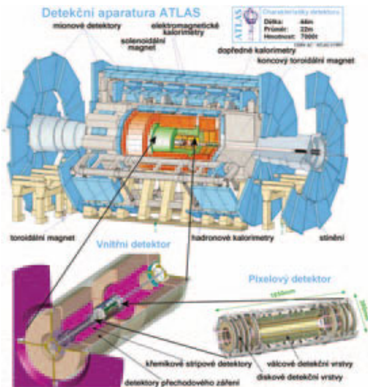
14/ Schéma detektoru ATLAS s umístěním centrálního dráhového detektoru
