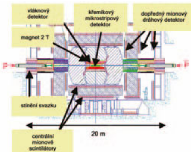
12/ Schematický průřez detektorem D0
