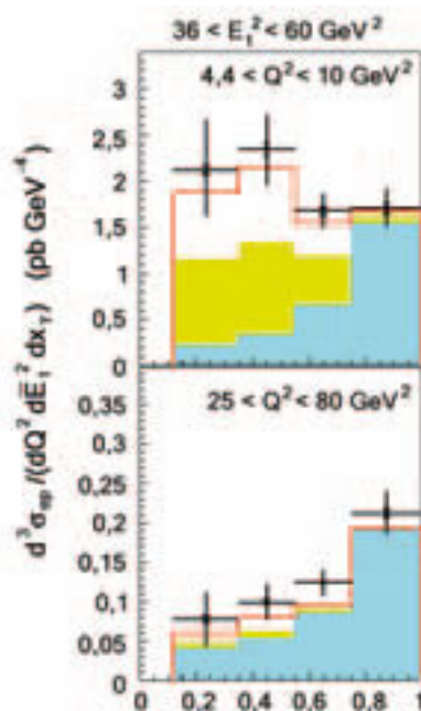
10/ Účinný průřez pro vznik dvou jetů ve srážce elektronu s protonem pro dva intervaly veličiny Q^2 . Modrý plný histogram představuje předpověď teorie bez započtení efektů struktury fotonu, červená čára po jejich započtení.
