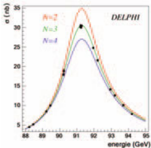
6/ Závislost účinného průřezu anihilace elektronů s pozitrony na hadrony dokazující, že existují právě jen tři generace fundamentálních fermionů.
