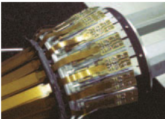
7/ Pixelový detektor DELPHI vyvinutý ve spolupráci s IHEP ve Vídni
