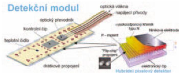
19/ Detekční modul detektoru ATLAS
