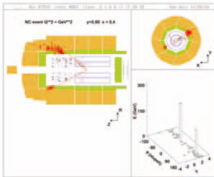
8/ Příklad srážky, při níž je rozptýlený elektron zaregistrován v elektromagnetickém kalorimetru (zelená část), a vyrážený kvark se v hadronovém kalorimetru (hnědá část) projevuje jako úhlově kolimovaný svazek částic. V levé části je podélný a v pravé horní příčný řez detektorem. V pravé spodní části je ve formě legoplotu vynesena závislost toku energie na azimutálním a polárním úhlu měřeném vůči směru primárního elektronu. Ačkoliv je jet tvořen mnoha částicemi, je tok energie podobný.
