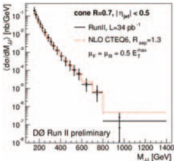
13/ Účinný průřez inkluzivní produkce dvojic jetů v závislosti na jejich invariantní hmotnosti.
