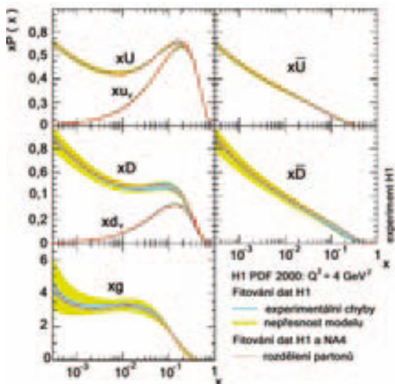
9/ Distribuční funkce kvarků U(x) a D(x) , antikvarků \bar{U}(x) a \bar{D}(x) a gluonů G(x) v protonu, získané z analýzy dat experimentů NA4 a H1. Všechny funkce jsou vynásobeny x .
