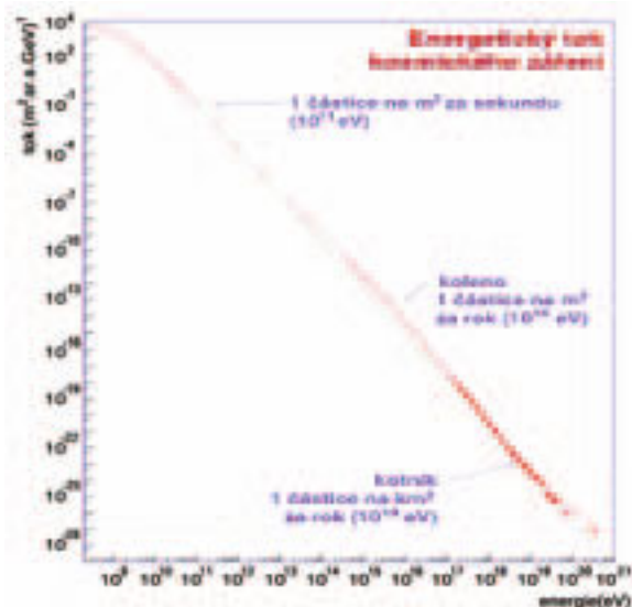
16/ Energetické spektrum kosmického záření
