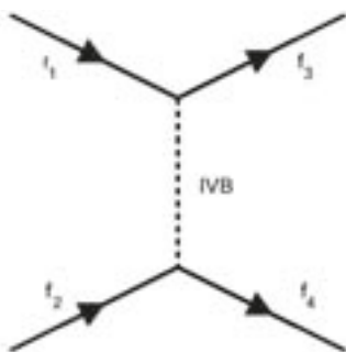
2/ Diagram znázorňující výměnný mechanismus sil působících mezi kvarky a leptony ( f_i ) ve SM
