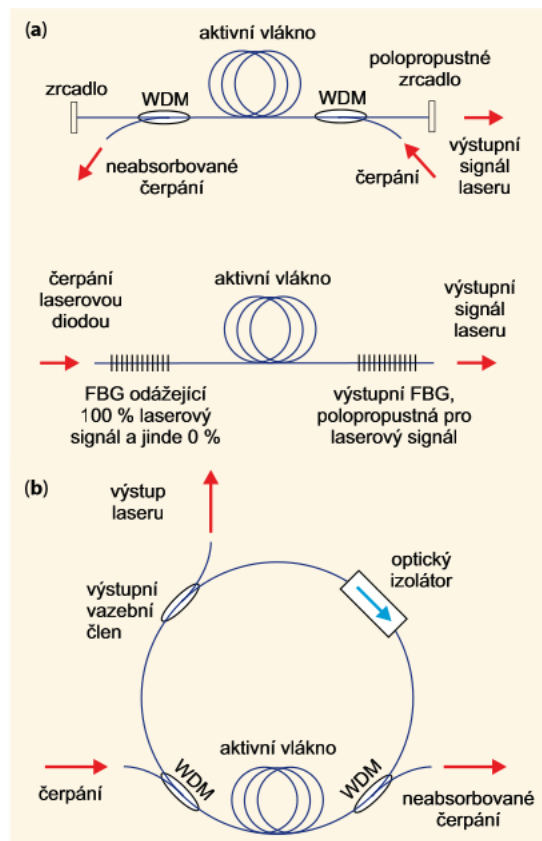
Obr. 1 Typická uspořádání vláknového laseru. (a) Fabryův-Perotův (lineární) rezonátor, (b) kruhový rezonátor.
