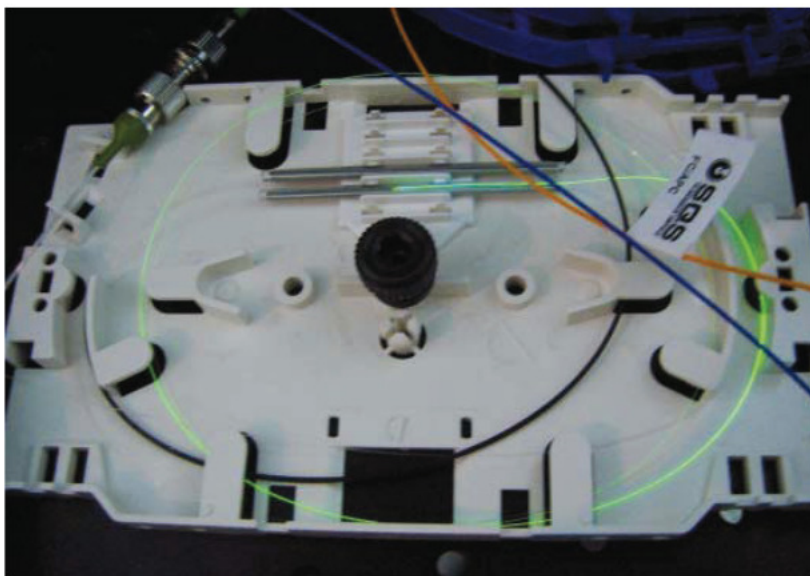
Obr. 4 Část femtosekundového laseru ze schématu na obr. 2b. V erbiem dopovaném vlákně je dobře patrná emise v zelené oblasti spektra, která je průvodním jevem ve vláknech vysoce dopovaných erbiem čerpaných na vlnové délce 980 nm.
