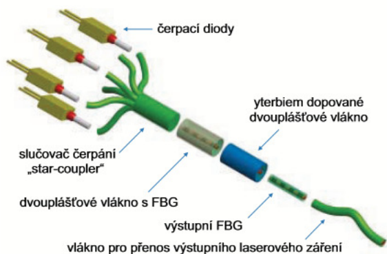
Obr. 6 Komponenty pláštěm čerpaného vláknového laseru.
