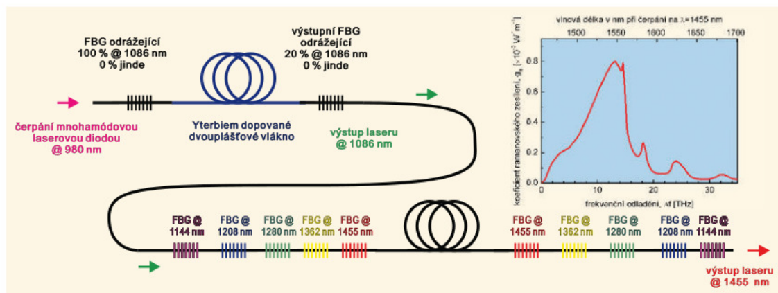
Obr. 9 Schéma ramanovského laseru používaného pro distribuované zesilování signálu v optických komunikacích. Vpravo nahoře je spektrální závislost koeficientu ramanovského zesílení pro standardní jednomódové vlákno.
