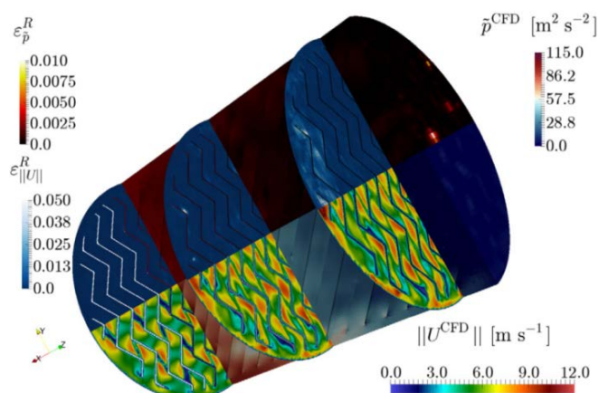
Obr. 12. Vyhodnocení shody původního CFD modelu a modelu redukovaného řádu pro proudění dusíku komplikovanou geometrií strukturované výplně destilační kolony.
