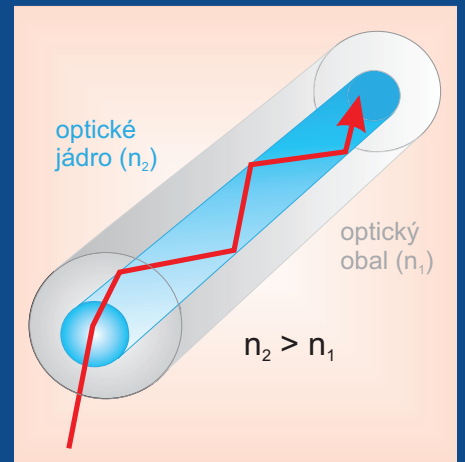
Obr. 3 Nahore: úplný odraz, vpravo: šíření světla v optickém vlákne.
