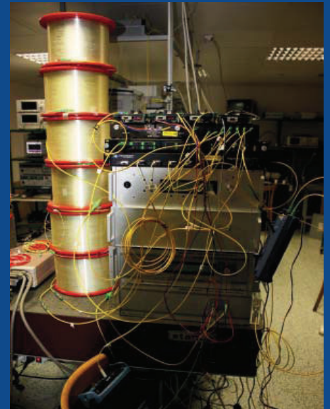
Obr. 11 Laboratorní měřicí pracoviště pro optický přenos signálů 10 \times 10 Gbit/s na 383 km optického vlákna navinutého na cívkách.
