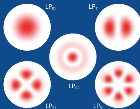
Obr. 5 Rozložení vidového pole.
