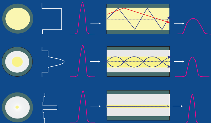
Obr. 6 Profily indexu lomu nejběžnějších druhů optických vláken (polymer-clad-silica, mnohavidové gradientní, jednovidové), popis šíření světla v těchto vlákních a deformace vstupních pulzů vlivem disperze a útlumu.
