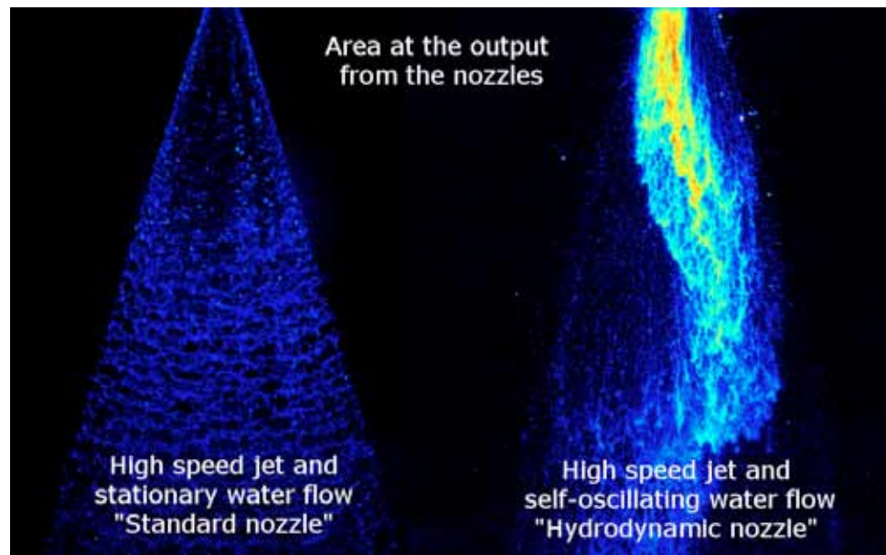
Vysokorychlostní paprsky vody na výstupu ze standardní a hydrodynamické trysky Vizualizace reálného proudění vysokorychlostních paprsků vody na výstupech ze standardní a hydrodynamické trysky.
