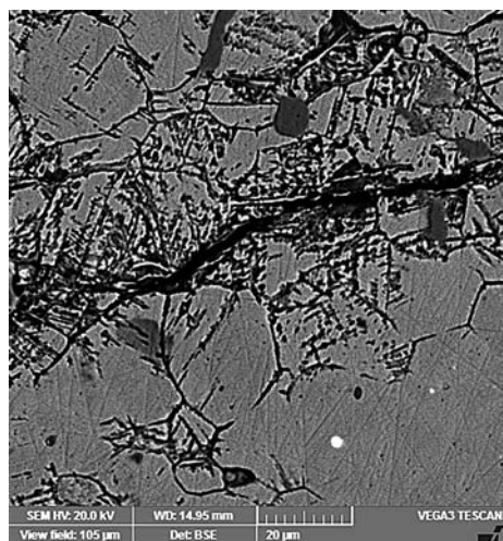
Obr. 5. Vzorek 1 bronzového pancíře. Korozní napadení bronzové slitiny podél hranic zrn a transkrystalické šíření trhlin v materiálu (šedé kulovité útvary jsou sulfidické vměstky).
