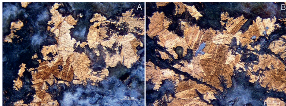
Obr. 4. Vzorek 1 bronzového pancíře. A: dvojčatění zrn a neorientované sulfidické vměstky ve velmi zkorodované bronzové matici (šedé útvary); B: dvojčatění zrn ve velmi zkorodované bronzové matici.
