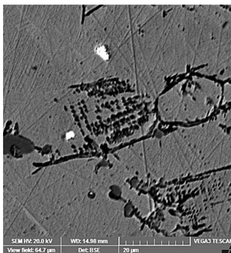
Obr. 6. Vzorek 1 bronzového pancíře. Částice olova a stříbra (světlé útvary).
