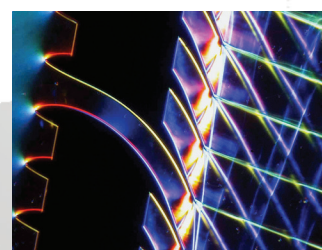
Barevný šlírový obraz proudění v modelu patního řezu oběžného kola posledního stupně parní turbíny velkého výkonu. Rychlost páry za modelem (na obrázku vpravo) je 1,9x vyšší než rychlost zvuku.
