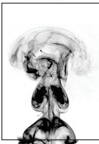
Kouřová vizualizace syntetizovaného proudu vzduchu.
