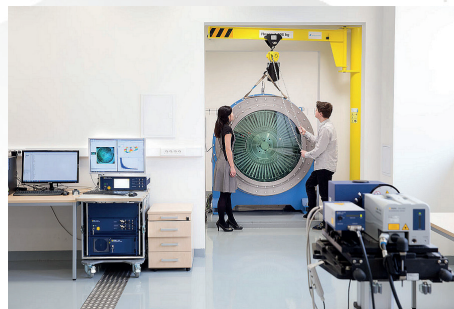
Laboratoř laserové rotační vibrometrie se zkušebním lopatkovým kolem.
