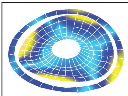
Vlastní tvar kmitů pryži odpruženého železničního kola.
