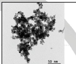
Platinové nanočástice pod elektronovým mikroskopem.
