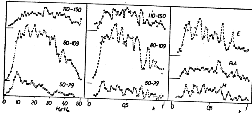
Fig. 2. A gauche: Fréquence de H_a - H_d (km) en fonction de l'altitude moyenne. Au milieu: Fréquences de k en fonction de l'altitude moyenne. A droite: Fréquences de k pour l'altitude moyenne 80-110 km en fonction de la saison de l'année. E = mai, juin, juillet, août; P + A = février, mars, avril, septembre, octobre; H = novembre, décembre, janvier.
