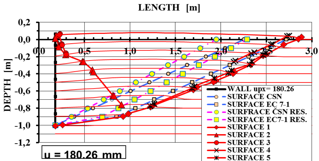
Experiment E5/0,3: Konečná analýza průběhu smykových ploch v tělese po rovnoběžném posunu čelní stěny (vlevo) o 180,26 mm. Čárkovně jsou vyznačeny smykové plochy podle současných teorií. Slabé červené čáry vyznačují svislé zdvihy v tělese.
