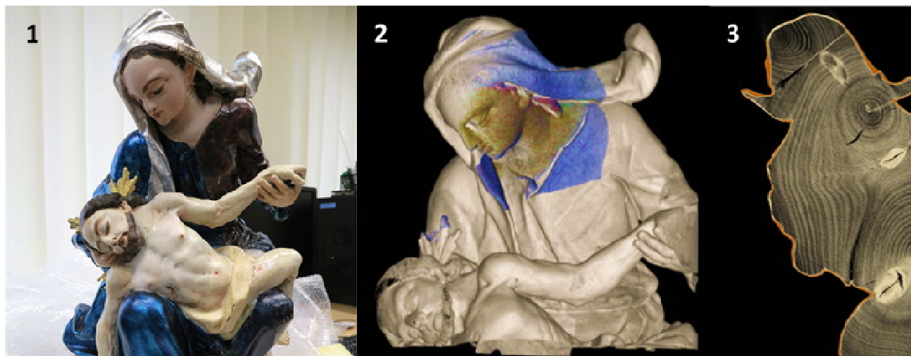
Výsledky sloučení XRF zobrazování prvkového složení povrchových vrstev s rentgenovou počítačovou tomografií popisující strukturu objektu
