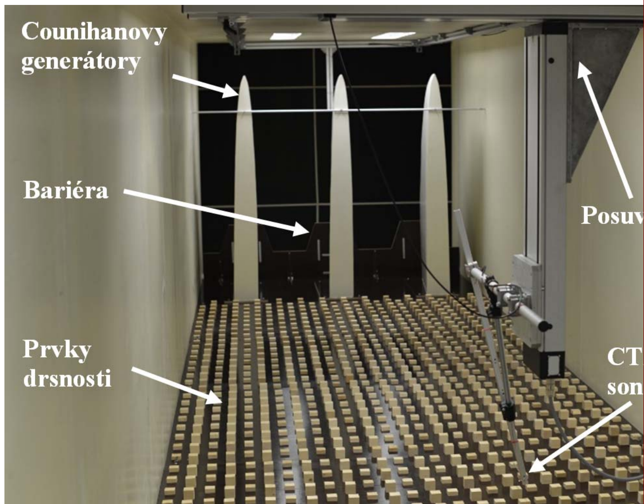
Prvky určené k modelování AMV v aerodynamické sekci Klimatického větrného tunelu.
