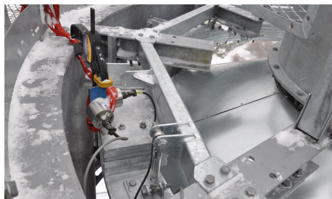
Obr. 3. Detail závěsů a jedné dvojice čidel. Foto: B. Přečová
