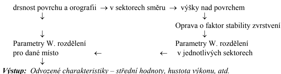
Schéma 2.2 Aplikace regionálních klimatologických charakteristik (Wind Atlas application model)
