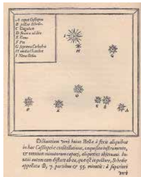
Termín „nova“ pro vzplanuvší hvězdu známe od dob Tychona Braha. Ten jej poprvé použil ve svém díle známém pod zkráceným jménem De nova stella vydaném v roce 1573.
