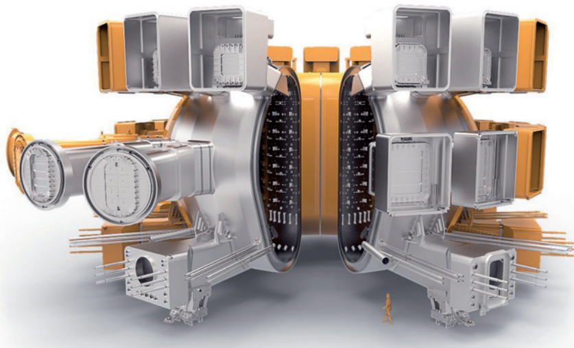
Obr. 16. Model vakuové nádoby ITER. Nádoba je dvouplášťová a je chlazená nebo ohřívána vodou s cílem udržení konstantní pracovní teploty. Pracovní teplota nádoby bude při experimentech 100 °C. Při vypékání (odplyňování) bude nádoba krátkodobě zahřátá na 200 °C [1]
