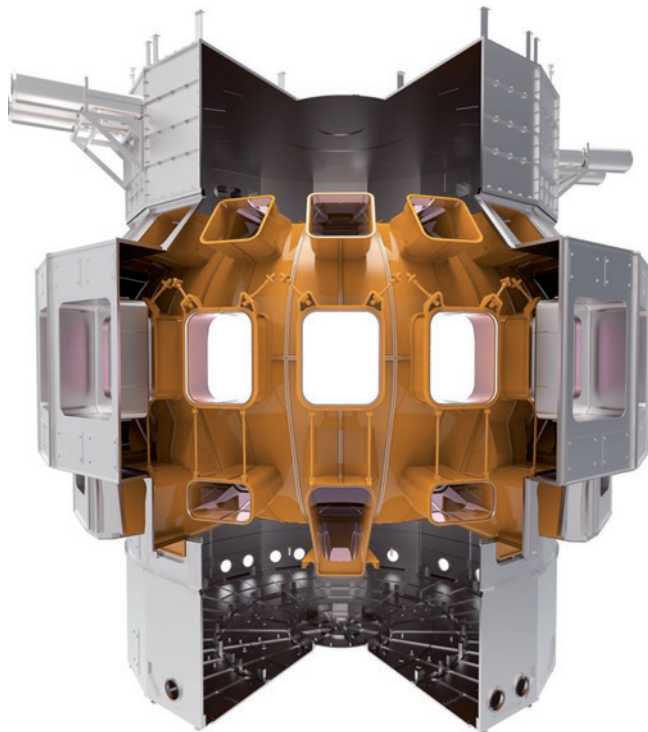
Obr. 20. Tepelný štít ITER bude chlazen plyným heliem o teplotě 80 K. Postříbřené nerezové panely sniží ohřev supravodivých cívek zářením [1]
