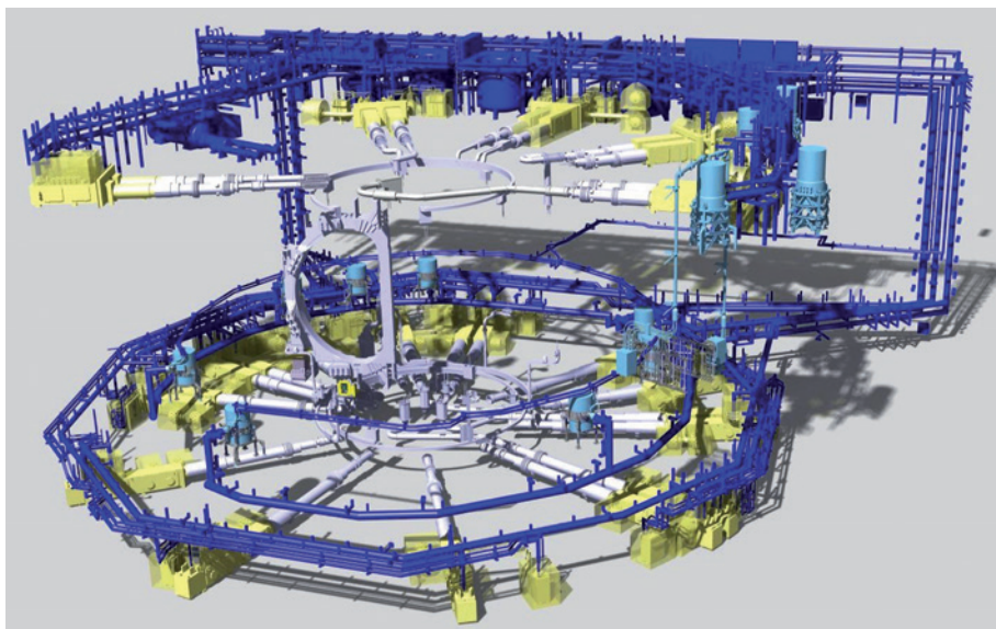
Obr. 19. Vizualizace distribučního systému kryogenního chladiva. Modře je zobrazeno rozvodné potrubí, světle modře kryoboxy. Žlutě a šedivě jsou zobrazeny přívody k supravodivým cívkám [1]
