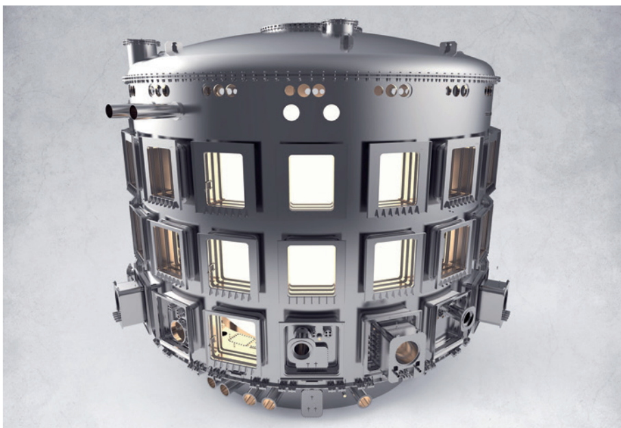
Obr. 17. Kryostat ITER bude po dokončení jedním z největších vakuových zařízení na světě. Jeho hlavním úkolem bude snížit tepelné ztráty supravodivých magnetických cívek pomocí vakuové tepelné izolace [1]
