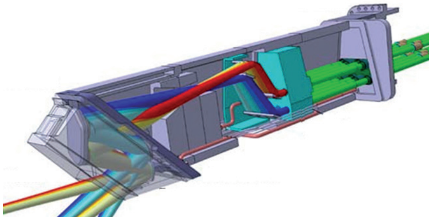
Obr. 28. Mikrovlnný zářič pro elektronový cyklotronový rezonanční ohřev ITER využitelný pro řízení plazmatu. Zářič umožňuje směřování mikrovlnného paprsku na různá místa v plazmatu [1]
