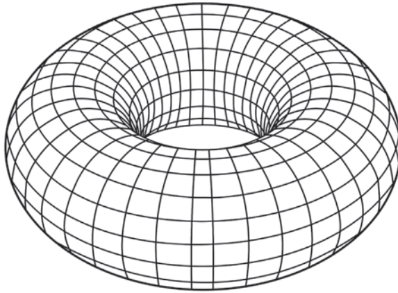
Obr. 10. Znázornění nehomogenity toroidální geometrie. Na vnitřním povrchu jsou čáry blíže k sobě než na vnějším povrchu
