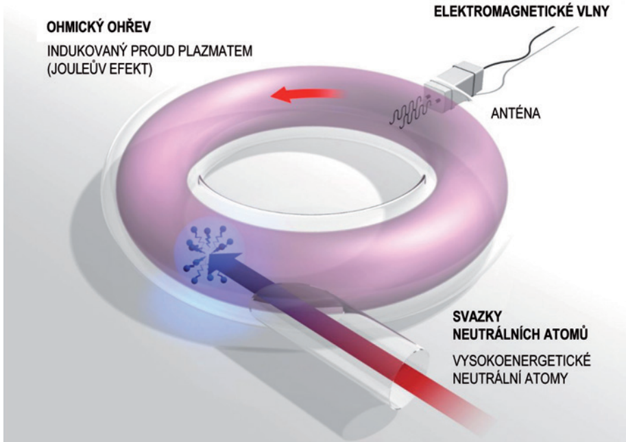
Obr. 23. Metody ohřevu plazmatu v tokamacích [1]
